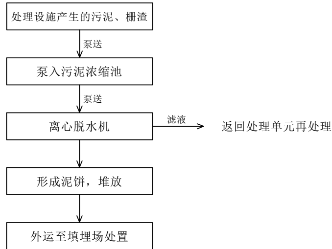
图 3-1 污泥处理工艺流程图
