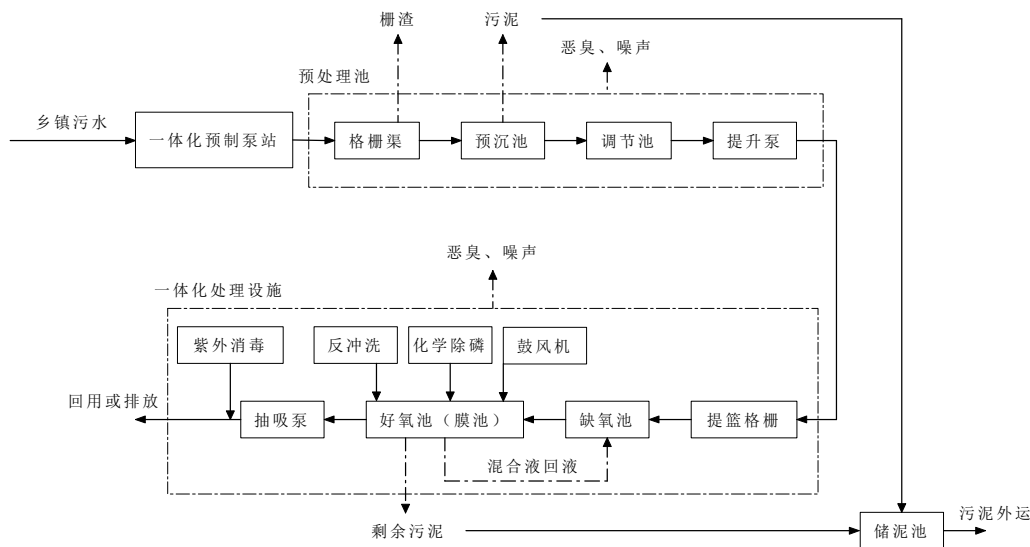
图 2-3 污水处理工艺流程及产污位置图
