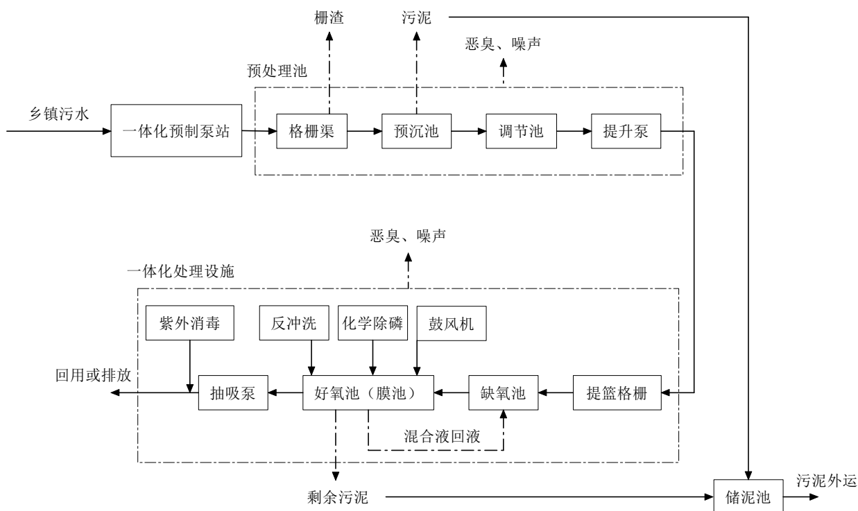
图 2-3 污水处理工艺流程及产污位置图
