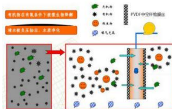
图 2-2 MBR 除污染物原理示意图
