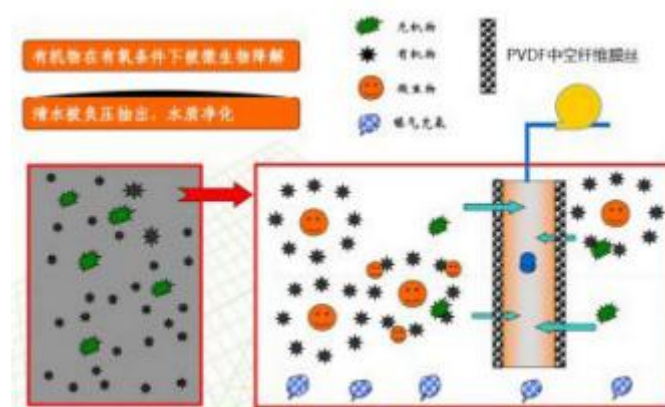
图 2-2 MBR 除污染物原理示意图
