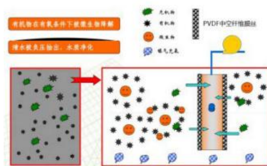
图 2-1 MBR 除污染物原理示意图
