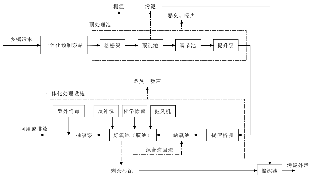
图 2-2 污水处理工艺流程及产污位置图
