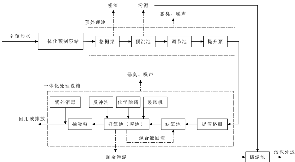
图 2-3 污水处理工艺流程及产污位置图
