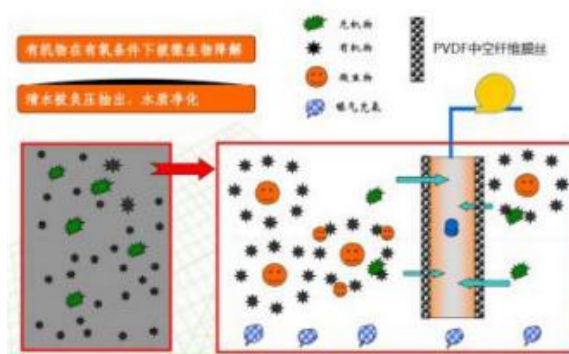
图 2-1 MBR 除污染物原理示意图
