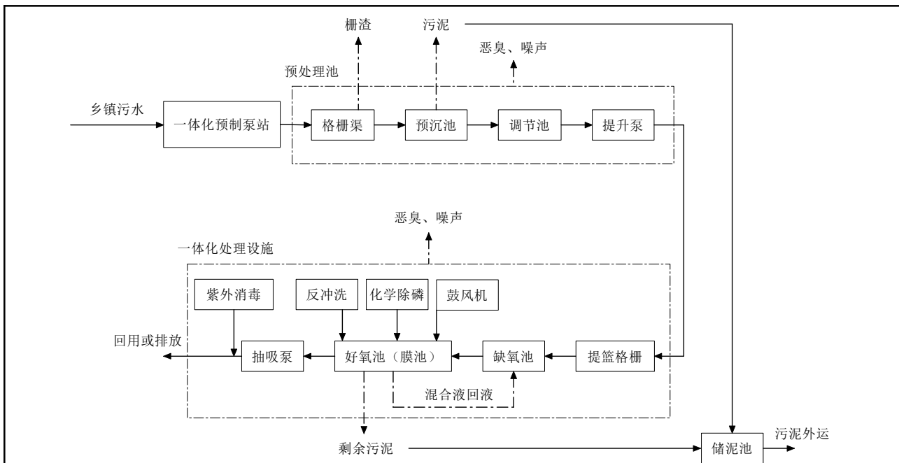
图 2-2 污水处理工艺流程及产污位置图
