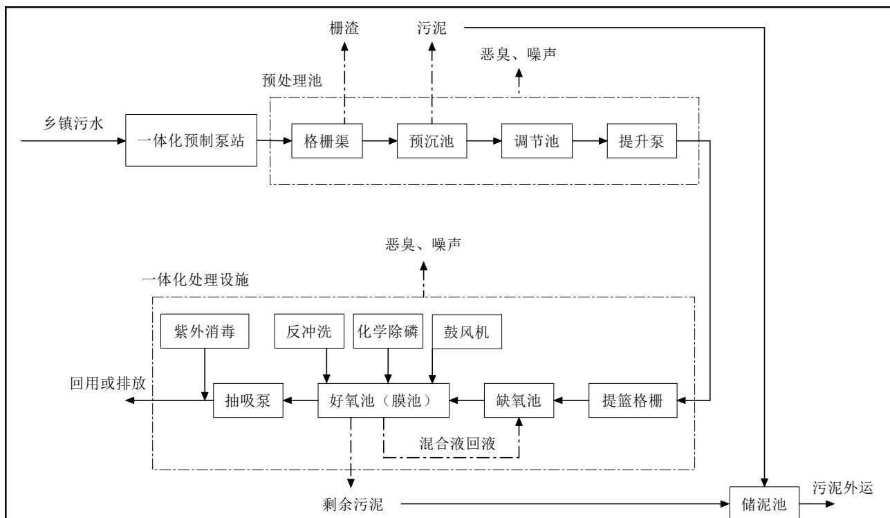
图 2-3 污水处理工艺流程及产污位置图
