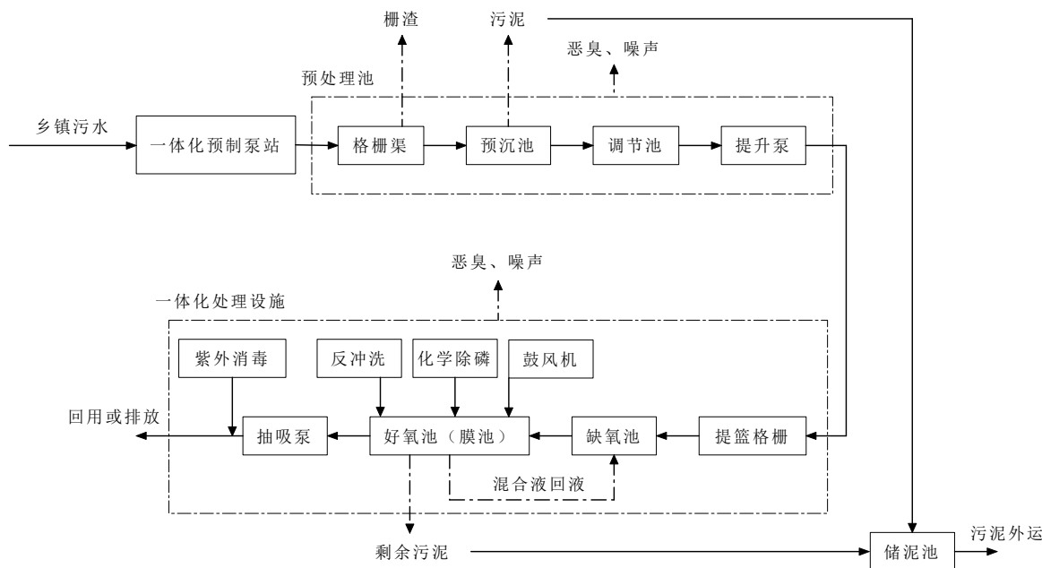
图 2-3 污水处理工艺流程及产污位置图
