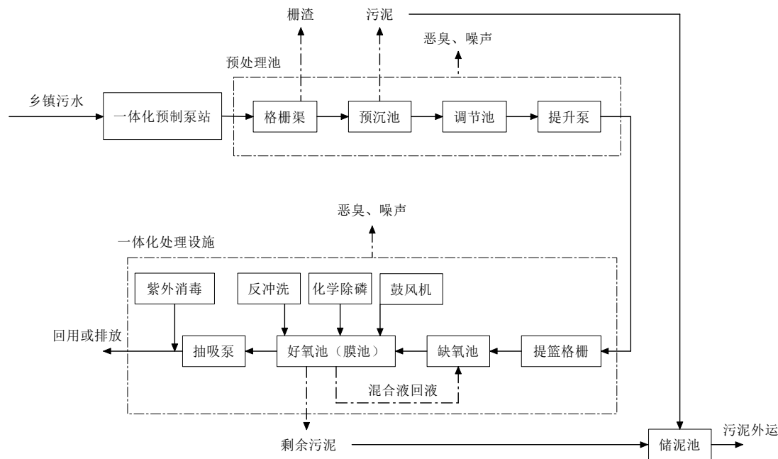
图 2-3 污水处理工艺流程及产污位置图
