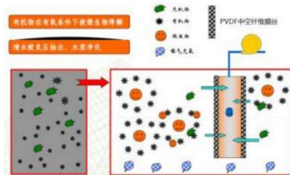
图 2-2 MBR 除污染物原理示意图
