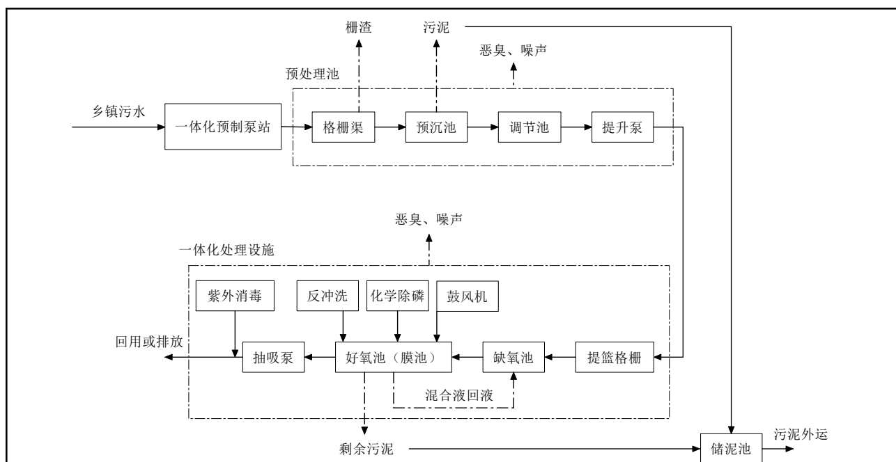
图 2-3 污水处理工艺流程及产污位置图
