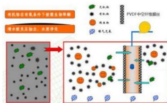
图 2-2 MBR 除污染物原理示意图
