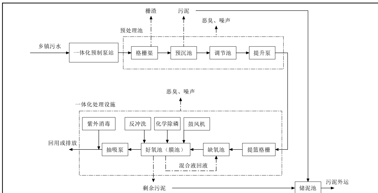
图 2-3 污水处理工艺流程及产污位置图
