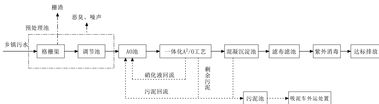
图 2-3 污水处理工艺流程及产污位置图
