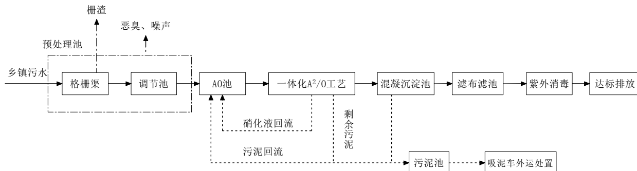
图 2-3 污水处理工艺流程及产污位置图
